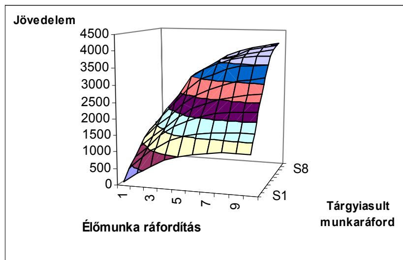
11. ábra. A célfüggvény értékének a változás az élómunka ráfordítás és a tárgyiasult munkaráfordítás (technikai színvonal), illetve általában kétirányú korlátozás változásának a függvényében.
