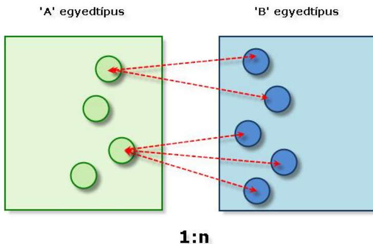
5. ábra 1:n
