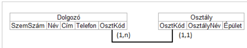
23. ábra Bachman-diagram
