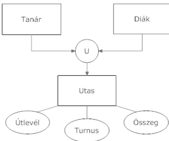
20. ábra Általánosítás
