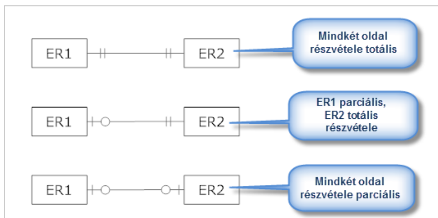
37. ábra 1:1 kapcsolatok
