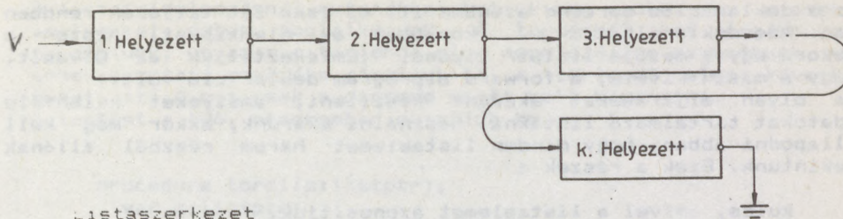
Listaszerkezet
