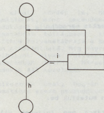
Ismétlési szerkezetek
