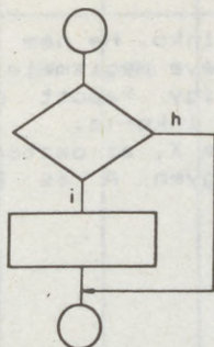
Kiválasztási szerkezetek
