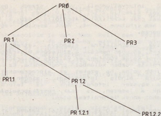
Hierarchikus programépítés
