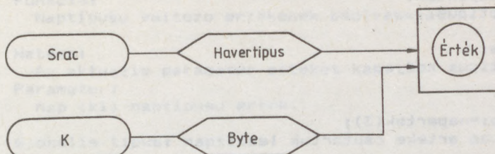
Álnév létrehozása
